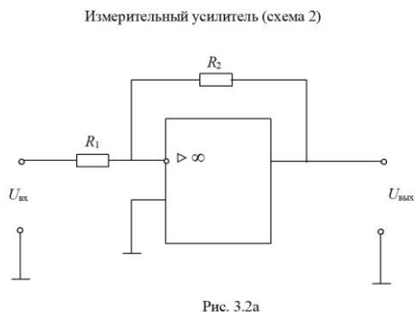
Figure 3 Схема измерительного усилителя 2.
