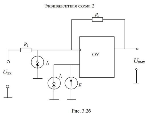
Figure 4 Эквивалентная схема ИУ2.
