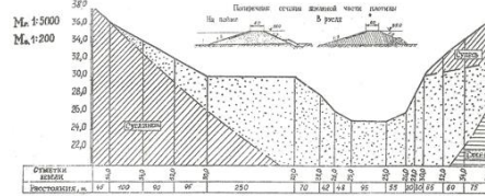
Поперечный профиль реки в створе гидроузла
