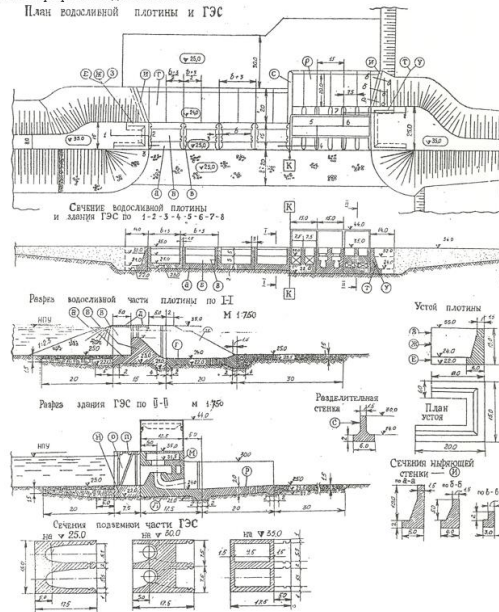
План и разрезы по зданию ГЭС и ВСП: План водоплавной плотины и ГЭС
