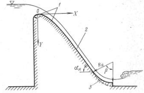
Рисунок 1 – Схема водобросной плотины: 1—водосливной оголовок; 2—сливная грань; 3—участок плавного сопряжения (пунктир) или сопряжения с уступом-трамплином (сплошная линия)
