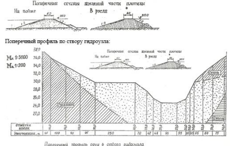
Поперечный профиль реки в створе гидроузла
