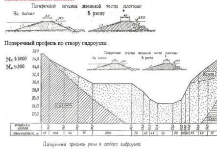
Профили грунтовой плотины:
