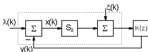
Рисунок 6.1. Обобщённая структурная схема следящей системы
