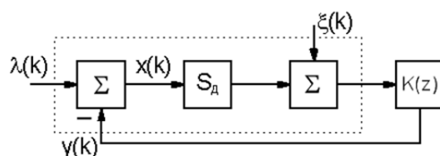
Рисунок. Обобщённая структурная схема следящей системы
