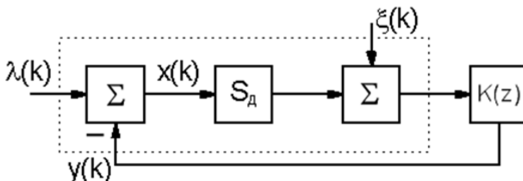
Рисунок . Обобщённая структурная схема дискретной СРА.
