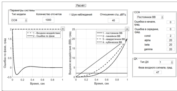
Рисунок 2. Интерфейс модели системы слежения за фазой сигнала
