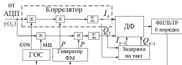
Рисунок 1. Схема дискретной нелинейной ССЧ
