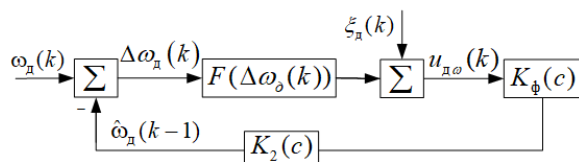
Рисунок 1. Схема дискретной нелинейной ССЧ
