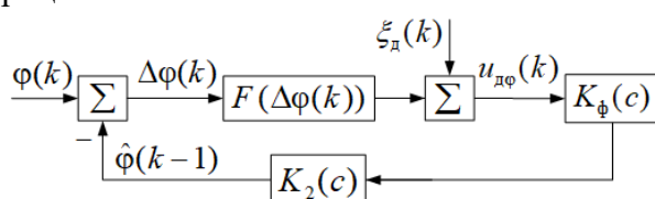
Figure 1 Рисунок 1. Структурная схема нелинейной дискретной ССЧ
