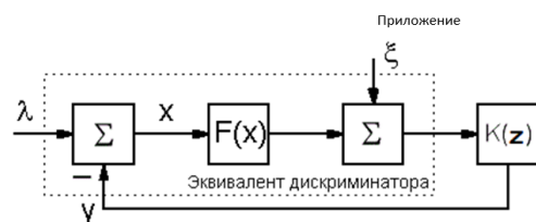
Рисунок 1. Структурная схема обобщённой дискретной системы радиоавтоматики
