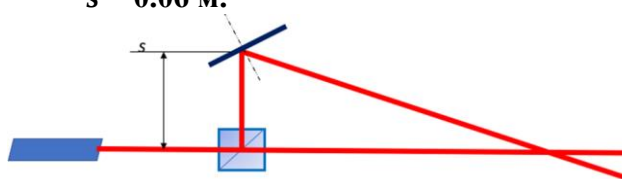
Figure 1 Интерференционная схема к задаче
