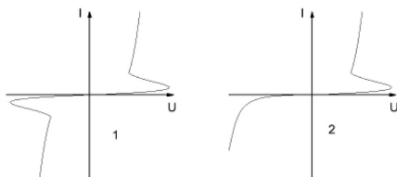
Figure 1 ВАХ тиристорной структуры
