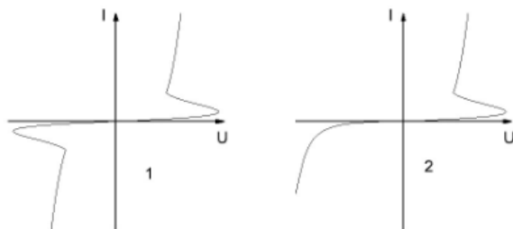
Figure 2 ВАХ тиристорной структуры
