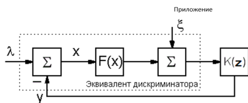
Рисунок 1. Структурная схема обобщенной дискретной системы радиоавтоматики
