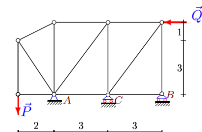
Figure 5 Найти усилия в стержнях
