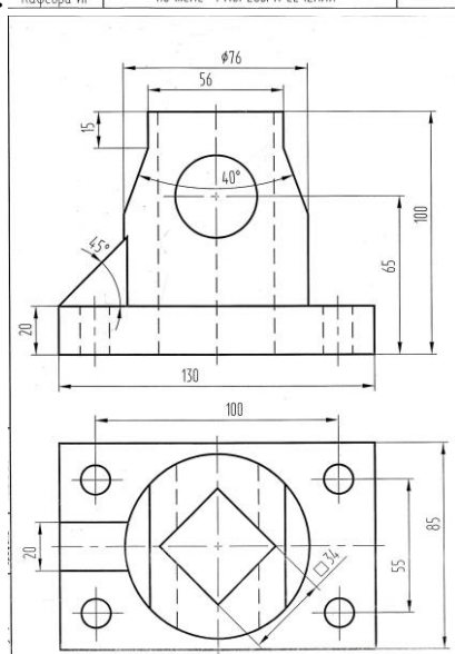
5. МЭИ (ТУ) Проверочная работа по теме "РАЗРЕЗЫ И СЕЧЕНИЯ" 1.60.25
