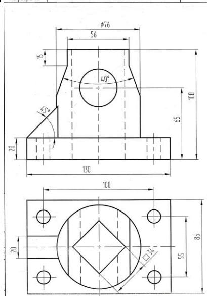
5. МЭИ (ТУ) Проверочная работа Кафедра ИГ по теме "РАЗРЕЗЫ И СЕЧЕНИЯ" 1.60.25
