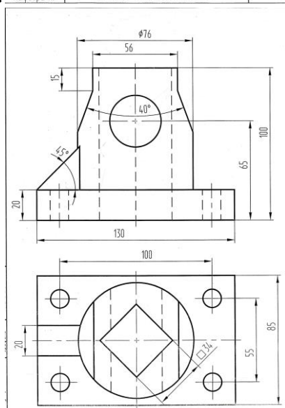
5. МЭИ (ТУ) Проверочная работа по теме "РАЗРЕЗЫ И СЕЧЕНИЯ" 1.60.25 Кафедра ИГ
