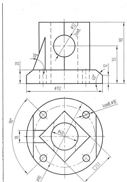
3. МЭИ (ТУ) Проверочная работа по теме "РАЗРЕЗЫ И СЕЧЕНИЯ" 1.60.23 Кафедра ИГ
