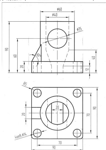
4. МЭИ (ТУ) Проверочная работа по теме "РАЗРЕЗЫ И СЕЧЕНИЯ" 1.60.24 Кафедра ИГ
