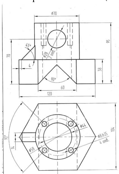
7. МЭИ (ТЧ) Проверочная работа Кафедра ИГ по теме "РАЗРЕЗЫ И СЕЧЕНИЯ" 1.60.22
