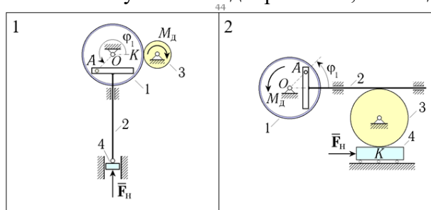
Figure 15 Схемы механизмов
