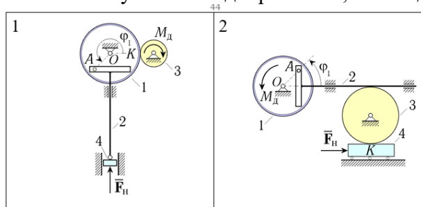
Figure 15 Схемы механизмов
