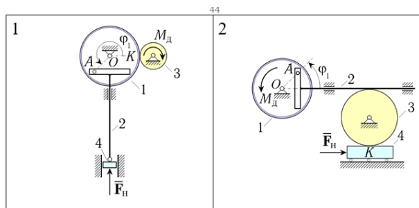
Figure 12 Схемы механизмов
