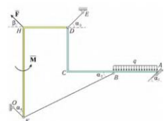
Рис. 1. Схема конструкции
