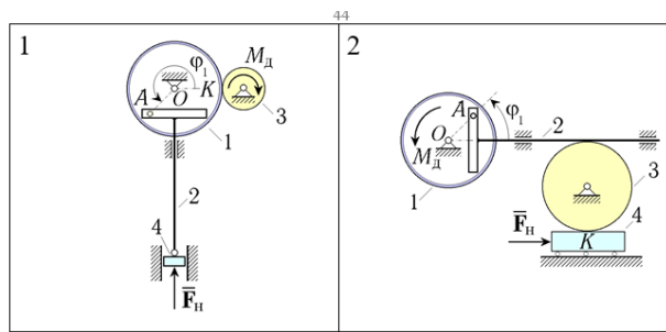
Figure 12 Схемы механизмов
