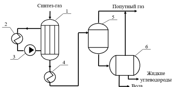
Figure 1 1- каталитический реактор 2 – теплообменник 3 – циркуляционный насос 4 – теплообменник 5 – сепаратор «газ-жидкость» 6 сепаратор жидких продуктов
