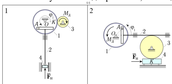
Figure 15 Схемы механизмов
