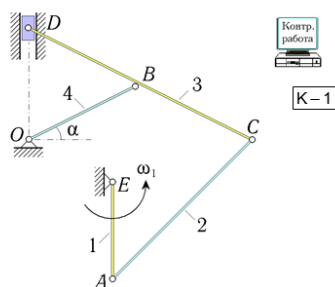
Figure 11 Вариант задачи контрольной работы "Кинематика плоских механизмов"
