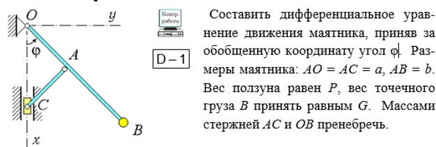
Figure 16 Вариант задачи контрольной работы "Составление уравнений динамики механизмов с одной степенью свободы в форме уравнений Лагранжа II-го рода"
