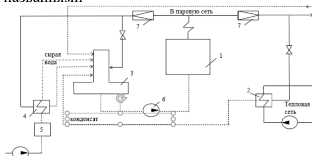
Figure 1 1 – паровой котел; 2 – сетевой подогреватель; 3 – деаэрактор; 4 – подогреватель химочищенной воды; 5 – блок химводоочистки; 6 – питательный насос; 7 – РОУ
