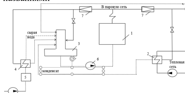
Figure 1 1 – паровой котел; 2 – сетевой подогреватель; 3 – деаэратор; 4 – подогреватель химочищенной воды; 5 – блок химоводоочистки; 6 – питательный насос; 7 – РОУ
