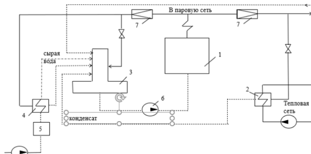
Figure 1 1 – паровой котел; 2 – сетевой подогреватель; 3 – деаэратор; 4 – подогреватель химочищенной воды; 5 – блок химводоочистки; 6 – питательный насос; 7 – РОУ
