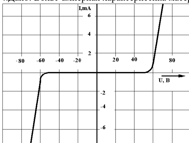
Рис. 1 Вольт-амперная характеристика варистора Рассчитать для U = 70 В:
