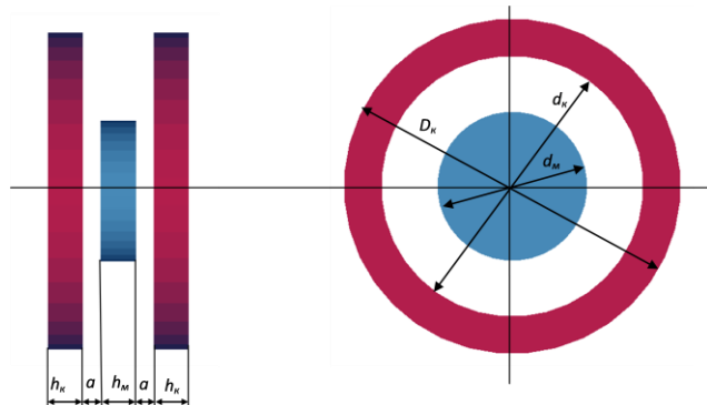
Figure 8 Геометрия магнитной системы
