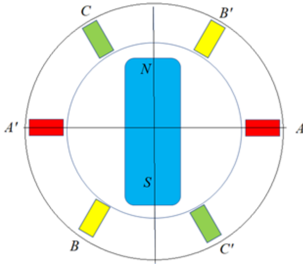
Figure 5 Схема генератора
