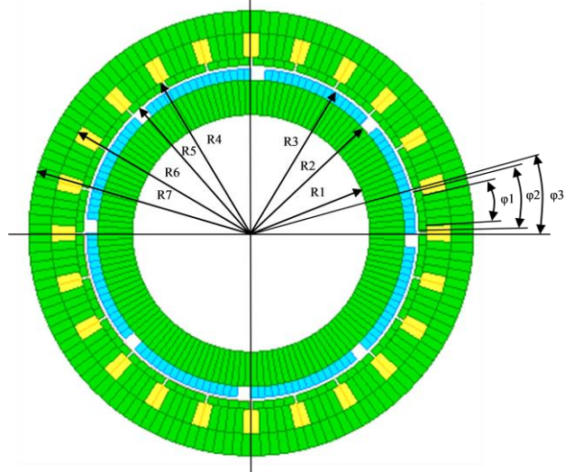
Figure 15 Геометрия магнитной системы
