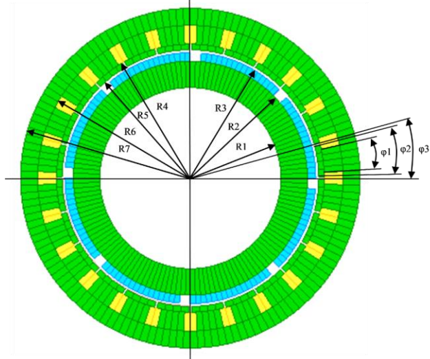
Figure 9 Геометрия магнитной системы
