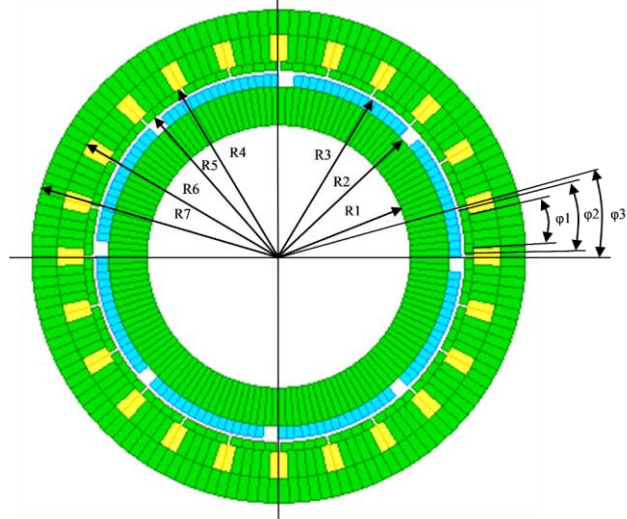
Figure 8 Геометрия магнитной системы
