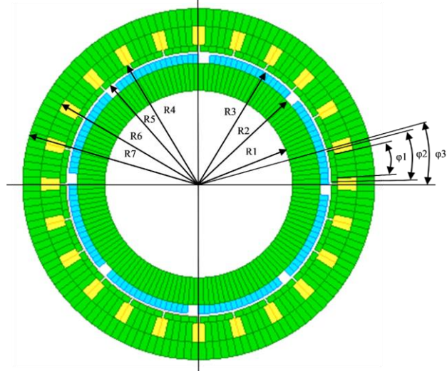
Figure 10 Геометрия магнитной системы
