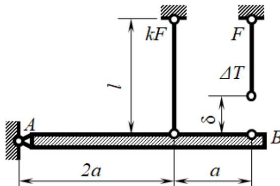
Figure 5 Расчетная схема проводников круглого поперечного сечения диаметром d рассматривается в виде системы стержней, изготовленных с отклонением от заданных размеров, причем начальный зазор \delta значительно меньше характерных размеров стержней. Найти монтажные силы и напряжения в проводниках после их сборки. Вследствие нагрева проводников при прохождении по ним электрического тока найти температурные силы и напряжения в проводниках, обусловленные перепадом температуры. Определить суммарные напряжения в проводниках и сделать вывод о прочности системы.
