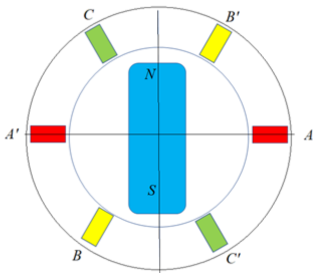
Figure 5 Схема генератора
