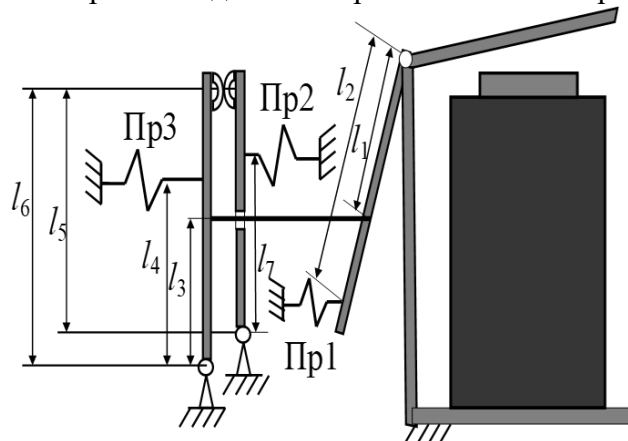
Figure 14 Кинематическая схема реле с РК
