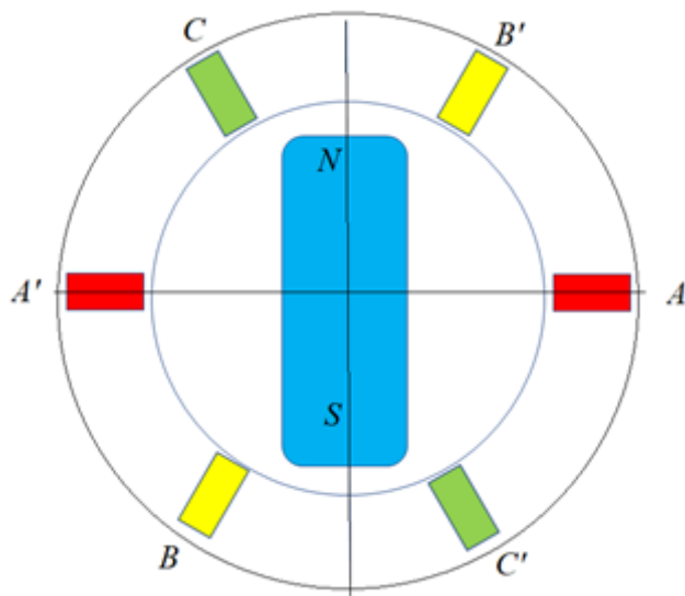
Figure 5 Схема генератора
