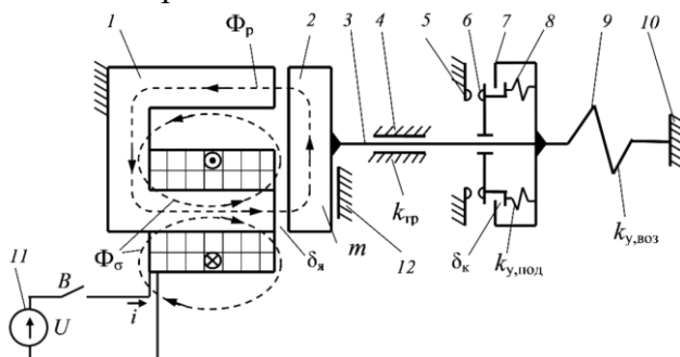
Figure 15 Кинематическая схема контактора постоянного тока
