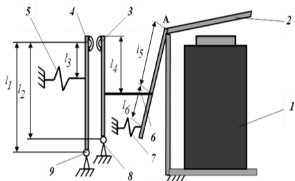
Figure 11 Кинематическая схема реле с ЗК
