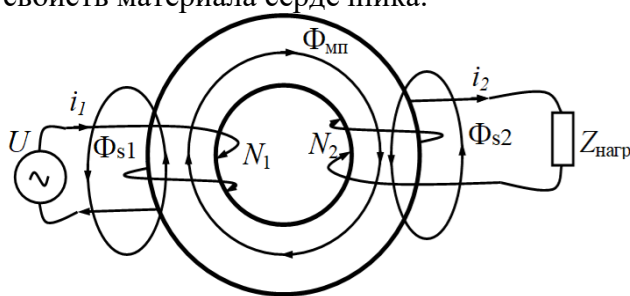
Figure 10 Схема трансформатора напряжения
