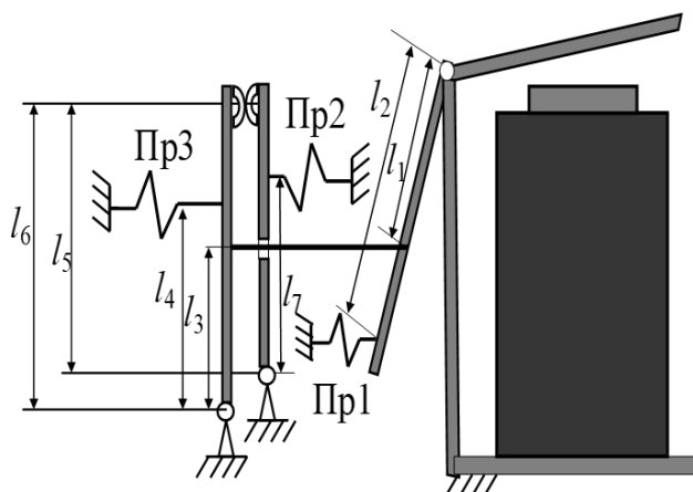
Figure 12 Кинематическая схема реле с РК
