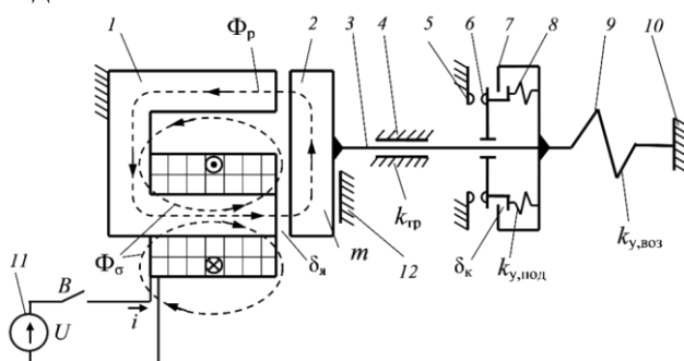
Figure 13 Кинематическая схема контактора постоянного тока
