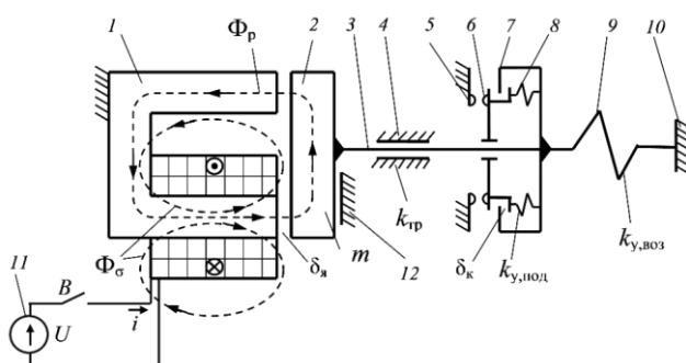
Figure 14 Кинематическая схема контактора постоянного тока
