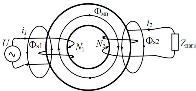
Figure 16 Схема трансформатора напряжения
