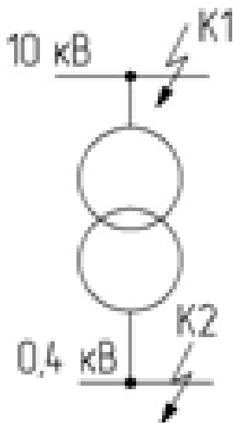
Figure 1 Цеховой трансформатор 10/0,4 кВ
