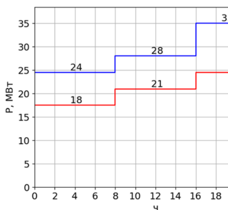
График нагрузки СН
