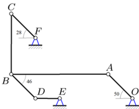
Figure 4 Рассчитать скорости механизма
