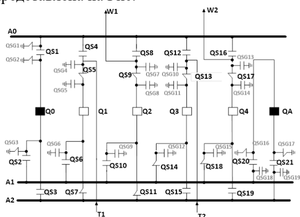
Рис. Нормальная схема работы РУ подстанции 110 кВ. Билет 10.
