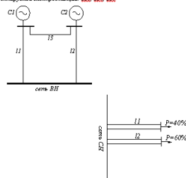
1.8. Принципиальная схема проектируемой электростанции: ТЗ, ТЗ, ТЗ
