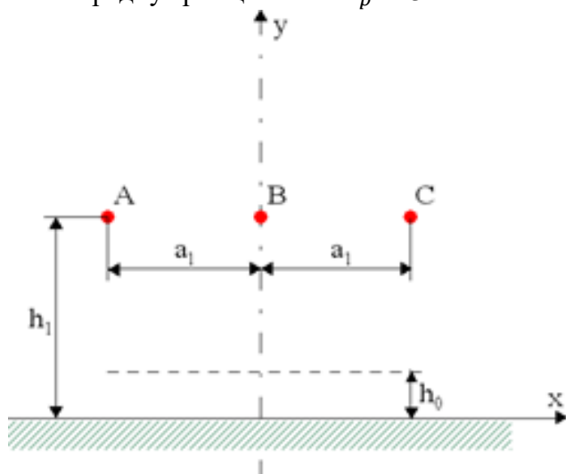
Рис. 3. К расчёту электрического поля под фазными проводами ВЛ с их горизонтальным размещением
