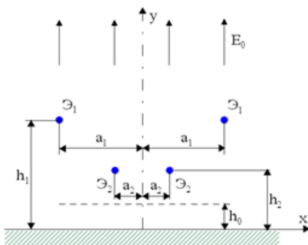
Рис. 6. К расчёту электрического поля под тросовым электростатическим экраном
