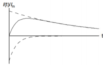
Figure 1 Рис. 1. Аппроксимация импульса тока молнии с помощью суммы двух экспонент
