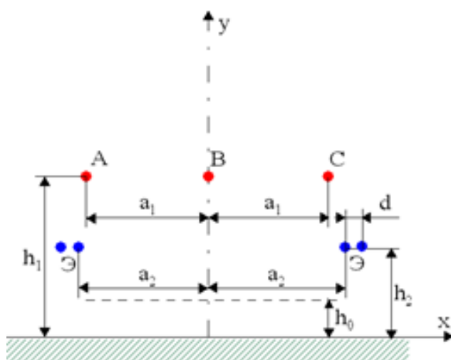
Рис. 2. Ограничение электрического поля ошиновки ОРУ 500 кВ под её крайними проводами
