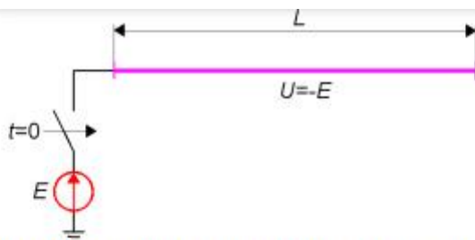
Рис. 3. К расчёту переходного процесса в длинной линии, вариант 3
