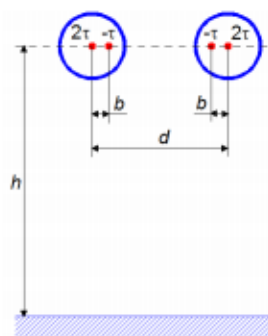
Figure 2 Рис. 2. К расчёту электрического поля одиночного фазного провода, расщеплённого на 2 составляющие
