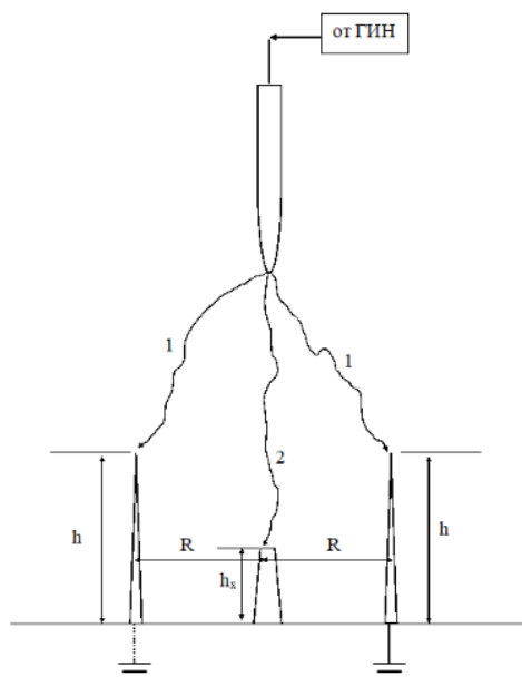
Figure 3 Рис. 3. Конфигурация электродной системы для раздела 1.2.2
