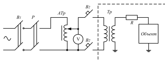
Figure 2 Рис. 2. Принципиальная схема установки.
