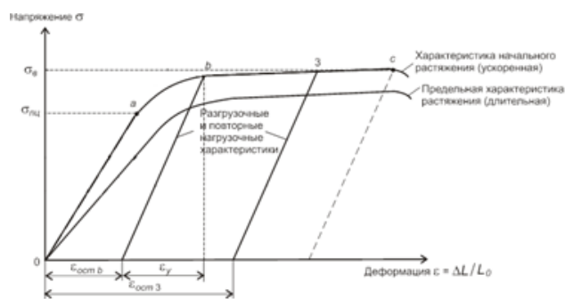
Figure 2 Рис. Экспериментальная диаграмма растяжения проволоки
