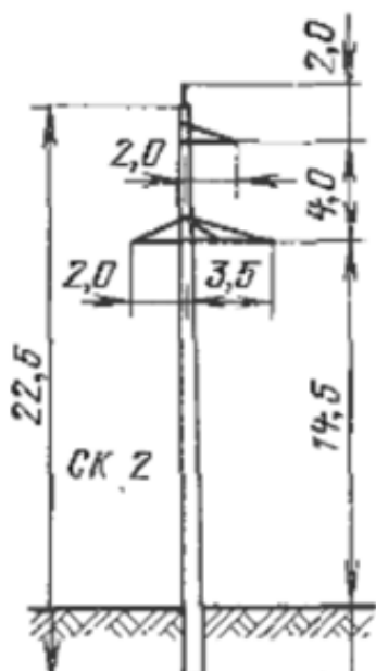
Figure 3 Рис. 1. Одноцепная промежуточная железобетонная опора ПБ110-5
