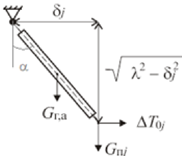
Figure 4 Рис. Равновесие поддерживающей гирлянды изоляторов
