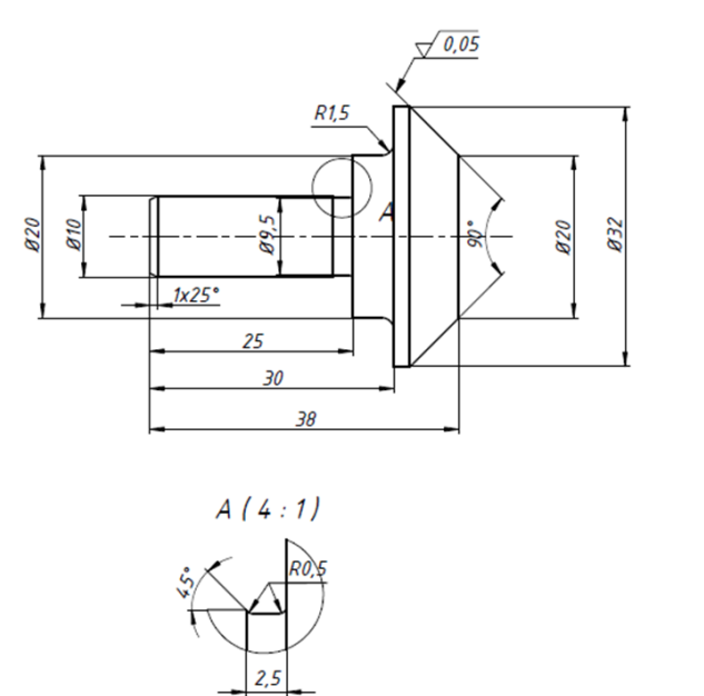
Figure 3 Клапан
