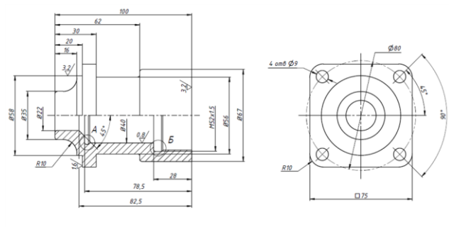
Figure 3 Клапан
