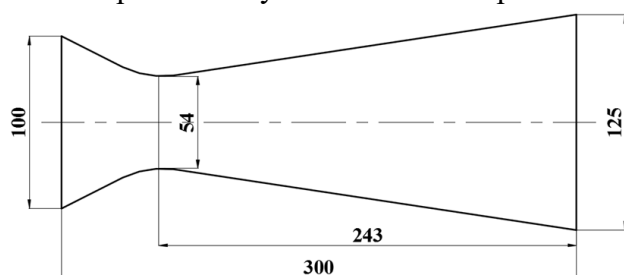
Figure 7 Геометрия исследуемого сопла Лавеля
